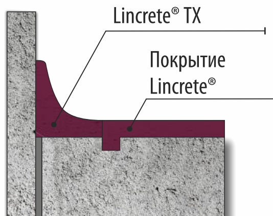
Примыкание к наружной стене
